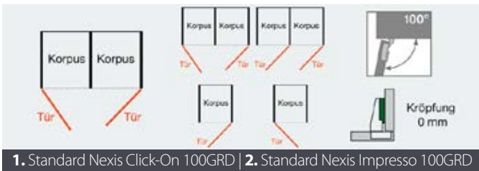
Scharnier mit Dämpfersystem
